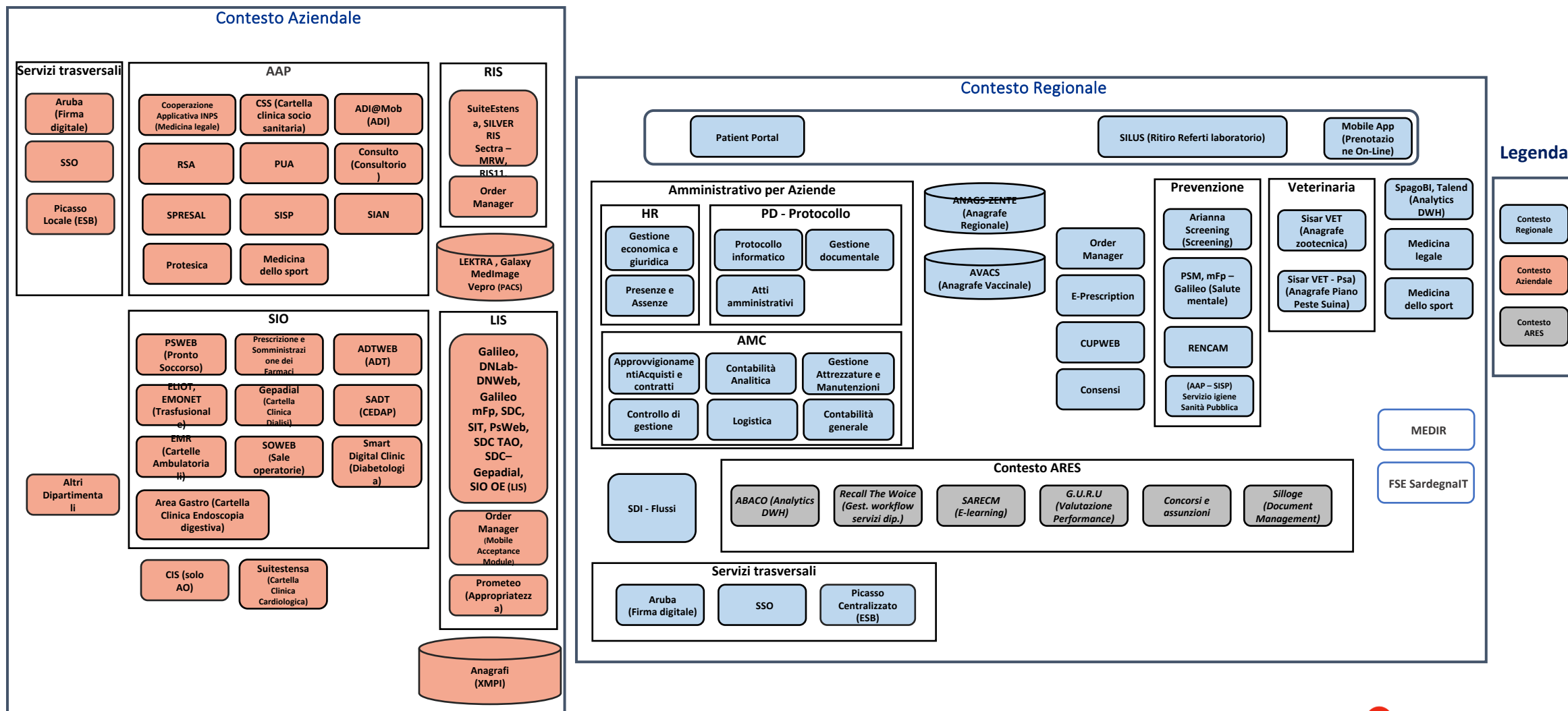
Figura 1. Schema concettuale complessivo dell'architettura regionale dei sistemi informativi per la Sanità
